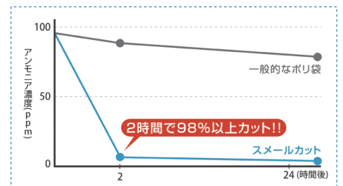
▲アンモニア臭の消臭速度 (添加剤メーカー製品研究所による調査に基づく)
