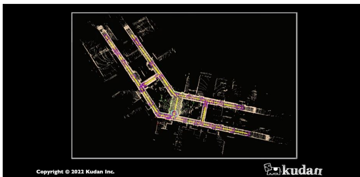
図 3 : Kudan の 3D-Lidar SLAM
