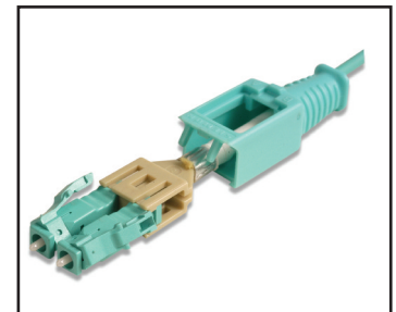
ラッチを180°回転させコネクタの極性を変更できる構造、ファイバやコネクタを捻ることが無くダメージを与えません。
