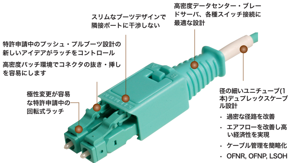
LC規格のアダプタとSFPモジュールに適合 (シャッター付きのアダプターには適合しません)
