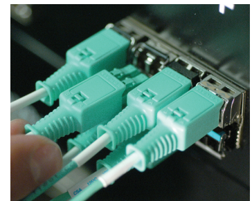
LC規格のアダプタとSFPモジュールに適合 (シャッター付きのアダプターには適合しません)
