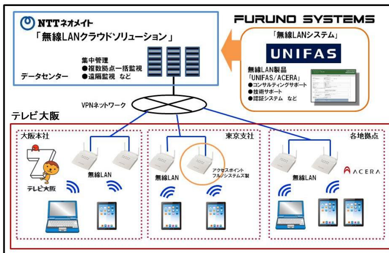
テレビ大阪 システム構成例
