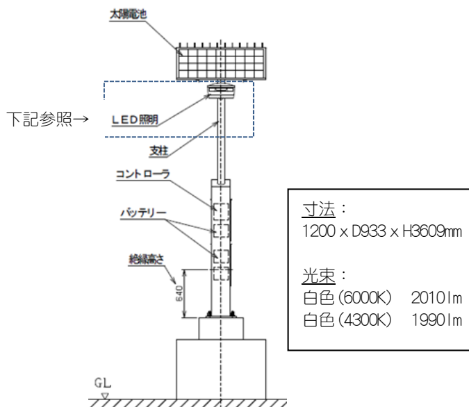
[図：ソーラー式 LED 照明の構成]
