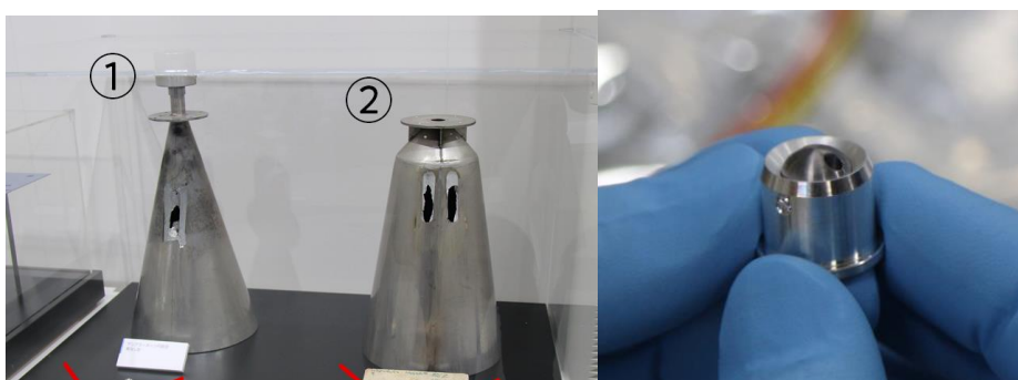
「はやぶさ」用サンプラホーン初期モデルと弾丸（写真 JAXA）
