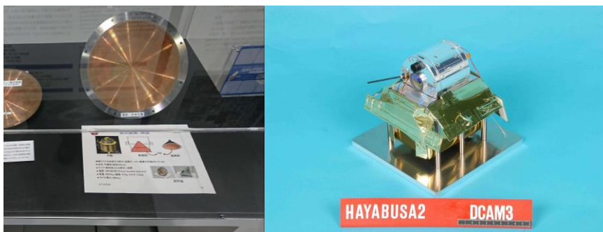
「はやぶさ2」搭載インパクターと分離カメラ DCAM3（エンジニアリングモデル） （写真：JAXA）
