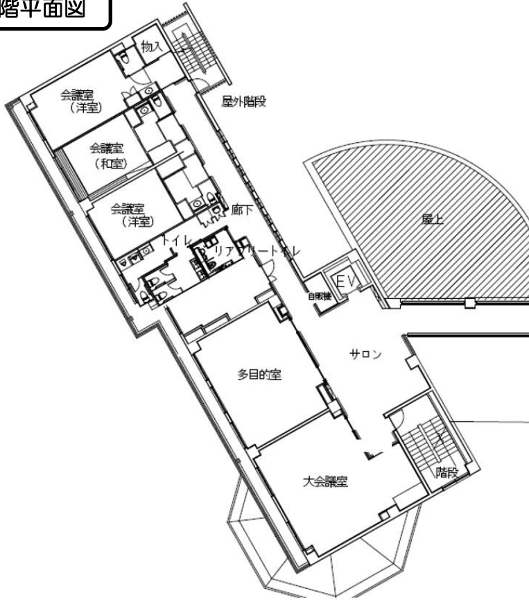
三和荘3階平面図
