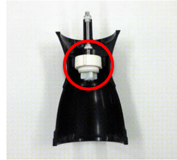
上下の臼を固定したフィックスグランド機構
