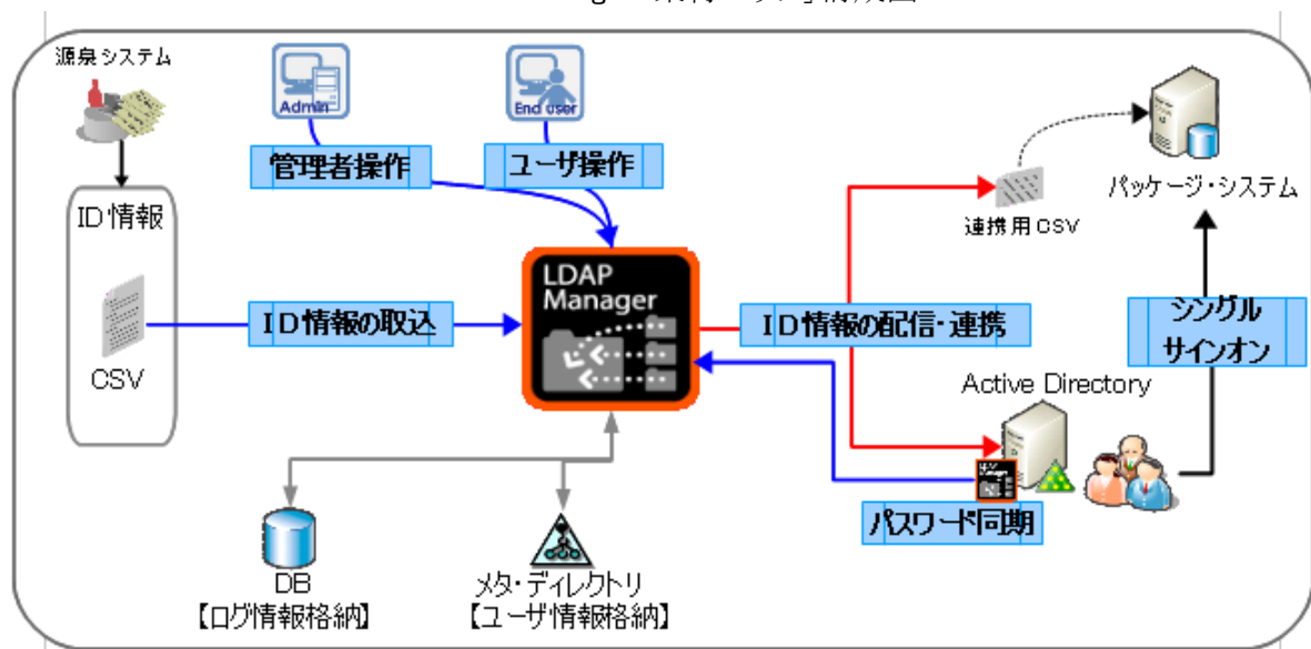
「LDAP Manager 楽得パック」構成図
