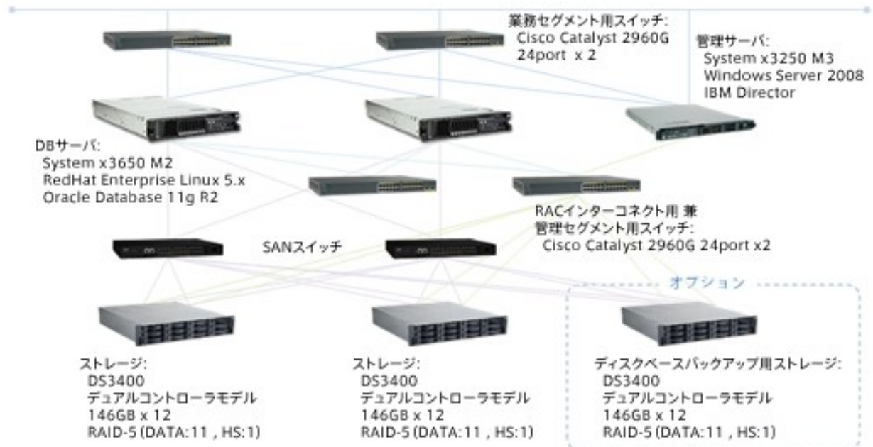
DODAI-i ストレージコスト削減モデル システム構成図
