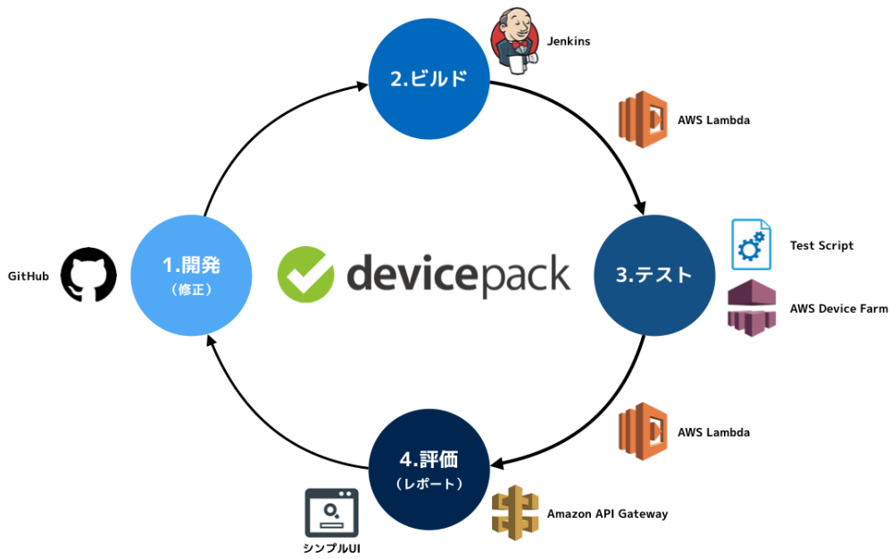
図 1 devicepack による動作テストの自動化イメージ
