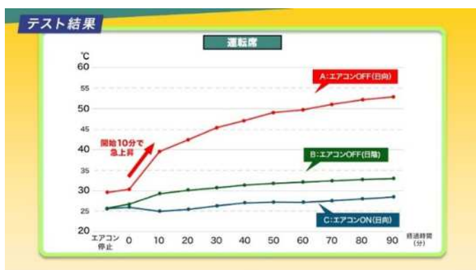
運転席の車内温度 推移比較
