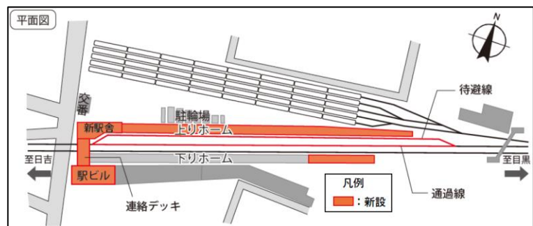
▲奥沢駅改修後イメージ(平面図)
