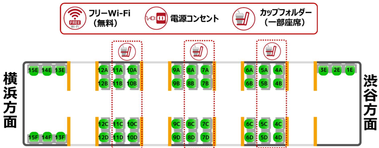
▲車両設備
