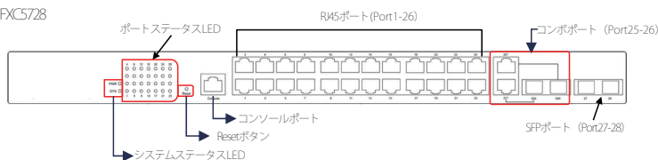
【前面図】
