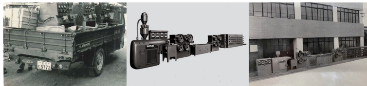
1950年代 押出機出荷風景 温度制御はスライダック方式
