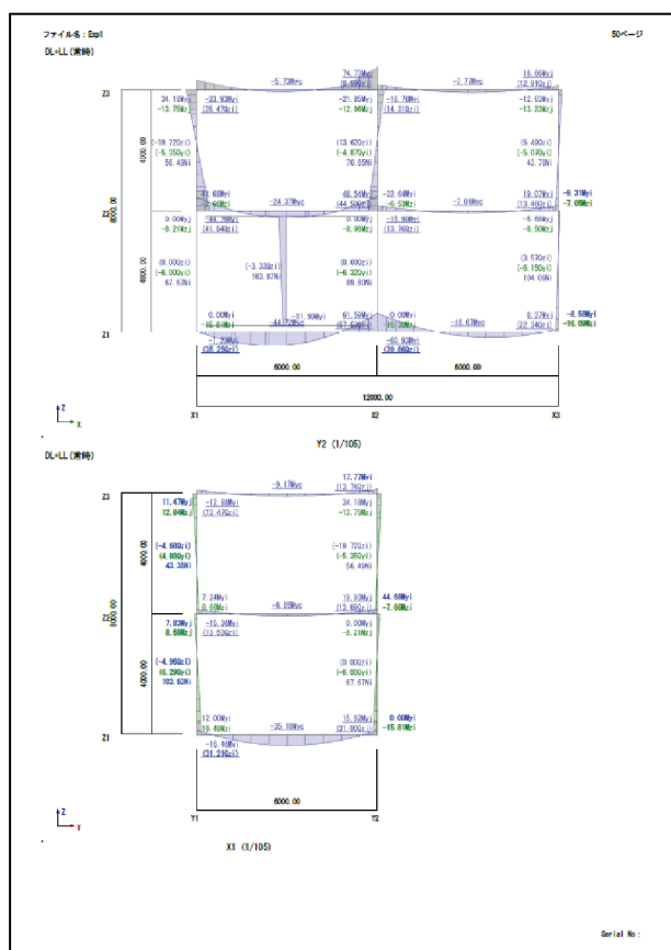
応力図と荷重図
