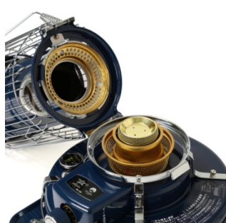
< 燃焼部 > ブルーフレームの特徴である青い炎が灯る部分です。
