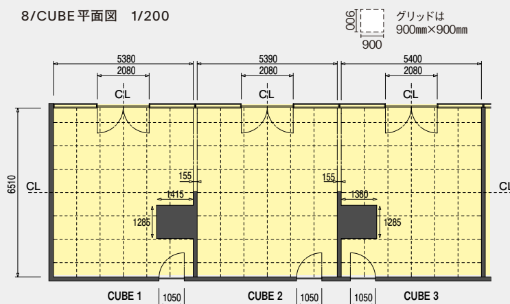
8/CUBE 平面図 1/200
