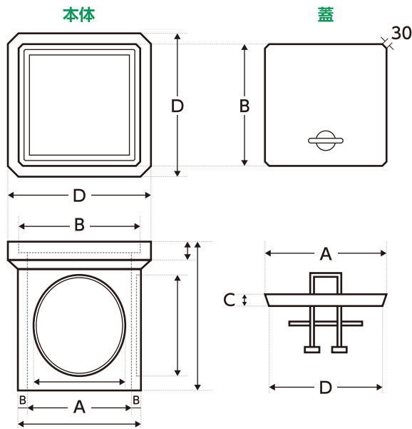
■寸法(mm)
