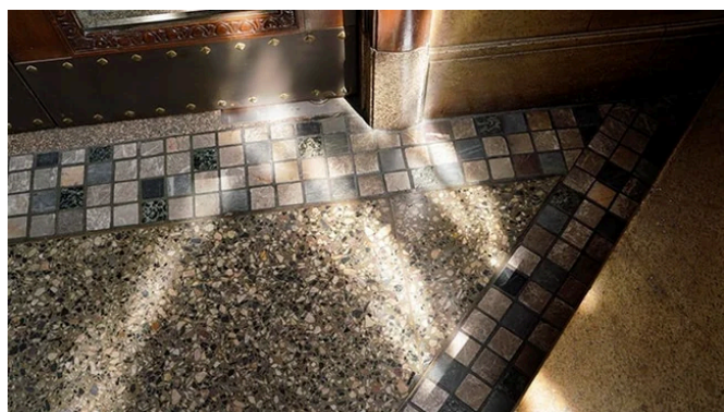
エントランスホール：石とテラゾー仕上げの組合せの床
