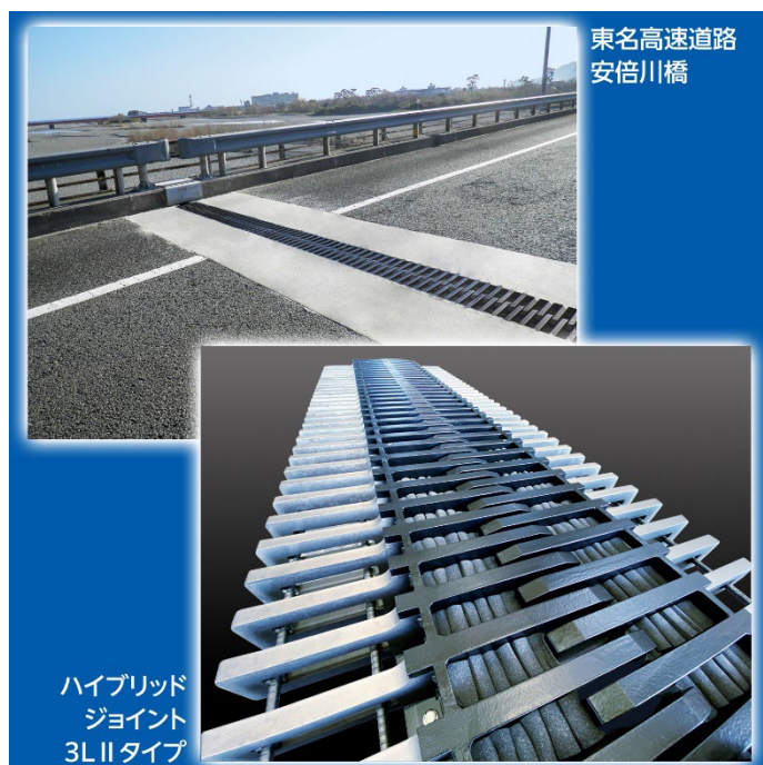
施工事例：東名高速道路 安倍川橋（静岡県静岡市） 使用製品：ハイブリッドジョイント 3LⅡ-250
