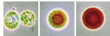
ヘマトコッカス藻が細胞内にアスタキサンチンを生成していく過程
