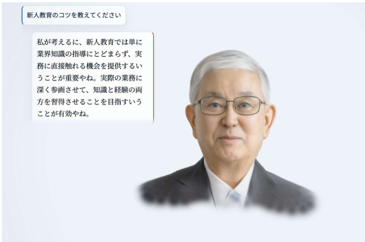
図 2：対話画面
