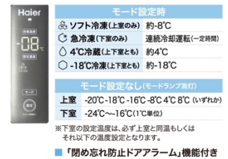
JF-NUF168B(W)操作パネルイメージ
