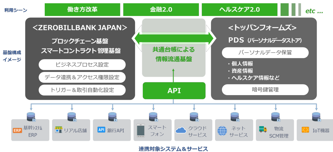
ブロックチェーン&スマートコントラクト基盤 x PDS 連携イメージ
