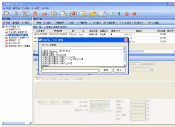
CSV フォーマット変換選択画面。 受注したデータは、各配送会社の送り状発行ソフトや、決済サービス用の CSV 形式でエクスポートできます。
