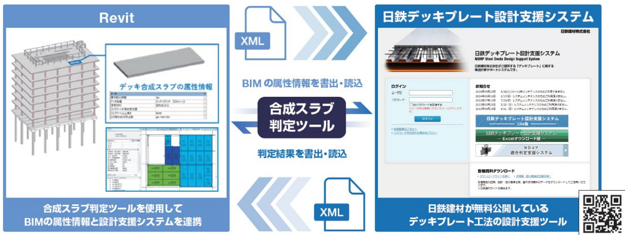
【合成スラブ判定ツールによる Revit と設計システムの連携イメージ】
