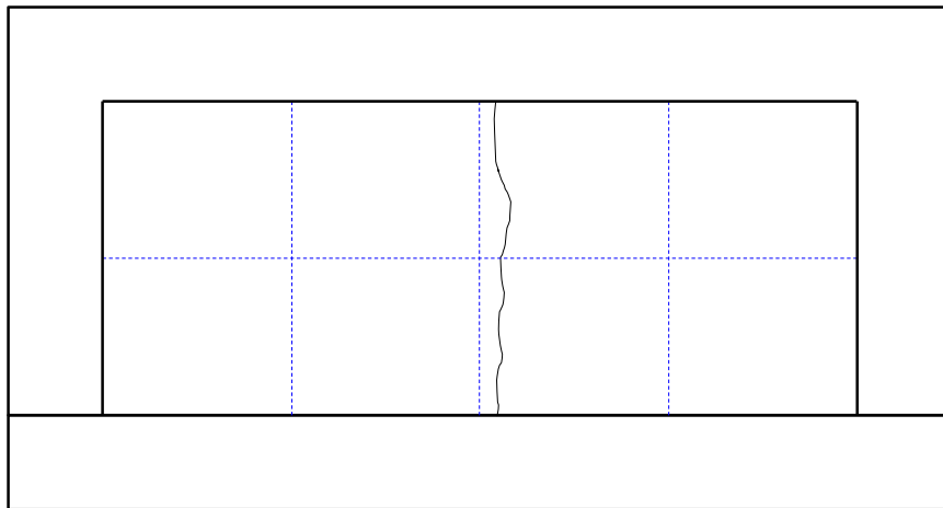
打設後 24 ヶ月の壁試験体の状況 【フィットクリート（高耐久クラス：目標収縮ひずみ 400 \times 10^{-6} ）】
