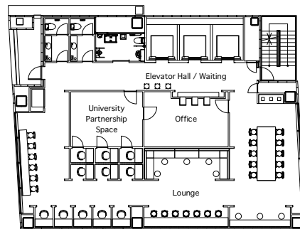
8F Plan
