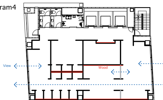
8F Plan
