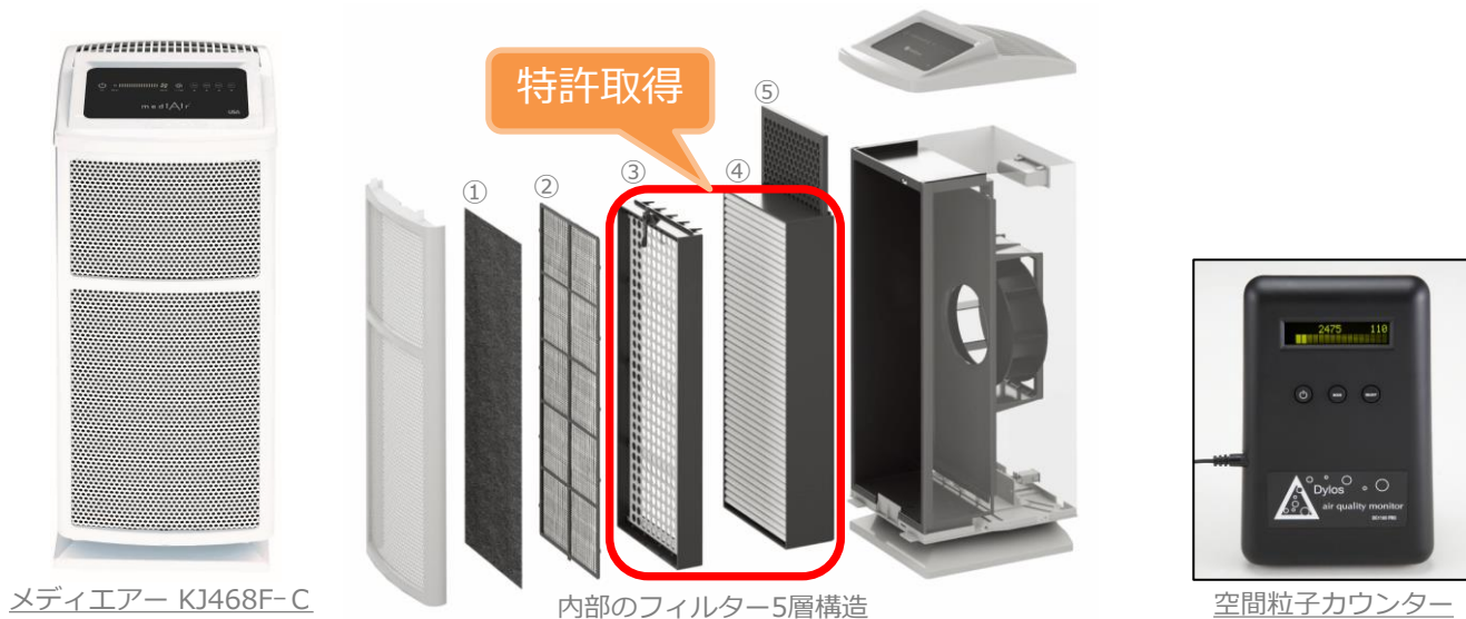
内部のフィルター5層構造
