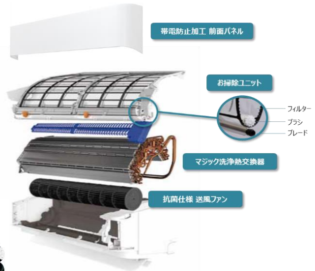
＜「プレミアムクリーン」構造イメージ＞
