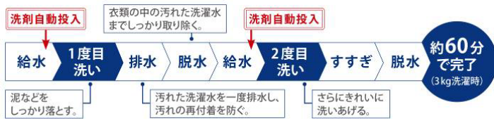
「自動2度洗いコース」の内容 ※TW-127X9において
