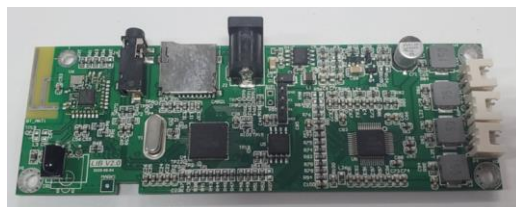
【Module-10/15 の外観】
