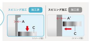
※：A：高さ A'：内筒の厚さ0.8mm A：加工前の内筒の厚さ3mm B：内筒の厚さ3mm C：ローラー
