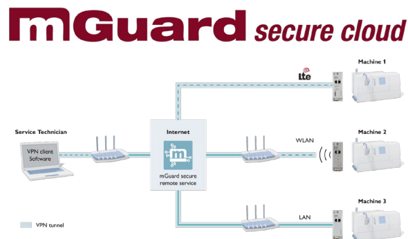
図2：mGuard Secure Cloudを介したリモートアクセス構成例
