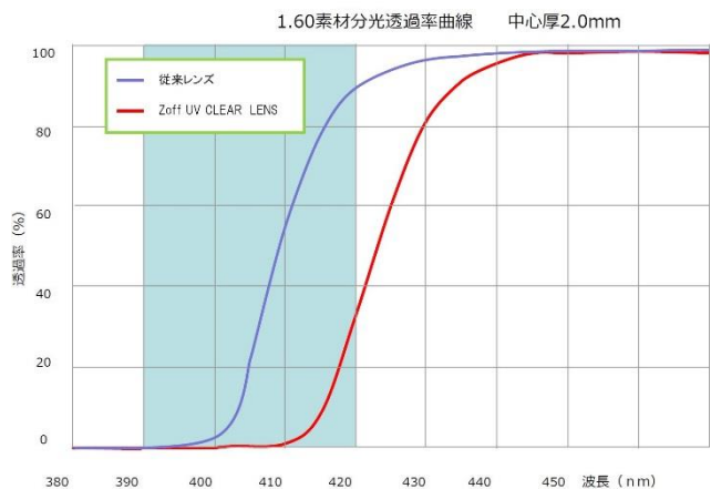
▲「Zoff UV CLEAR LENS」と従来のレンズのカット率を比較。本商品は 420nm までの光を高確率でカット※。
