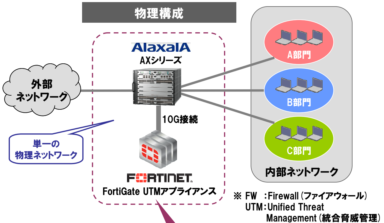
図1 ネットワーク・パーティションとVDMによるネットワーク構築例
