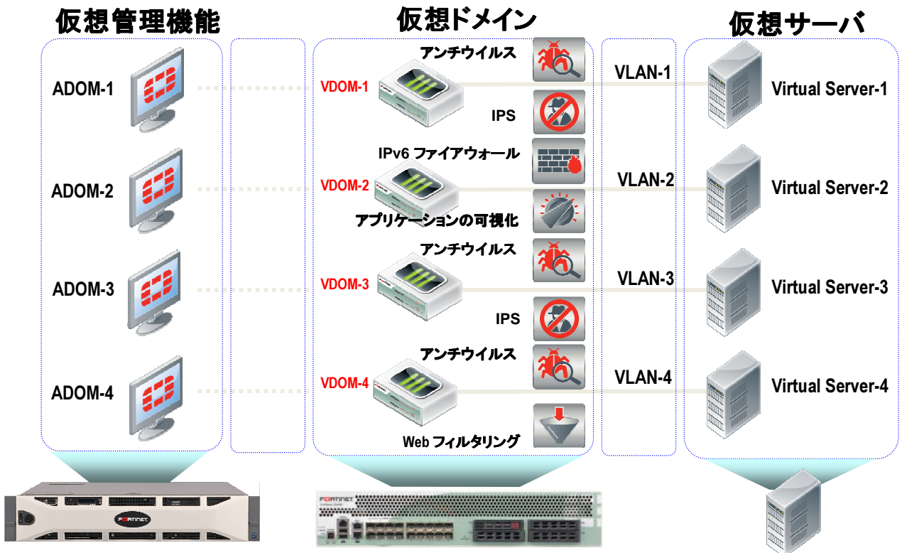
図3 仮想ドメイン(VDOM)論理構成例
