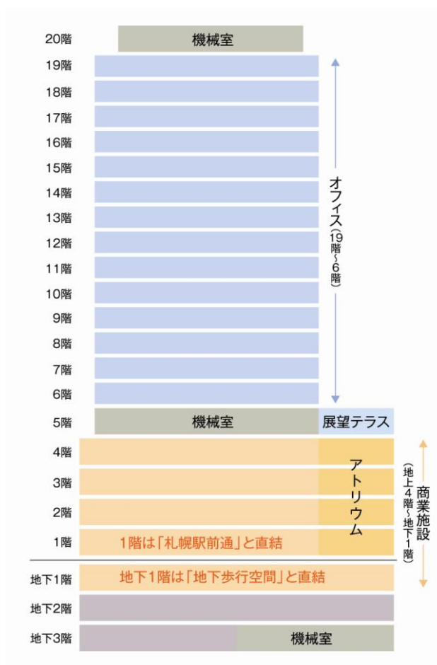
建物断面図
