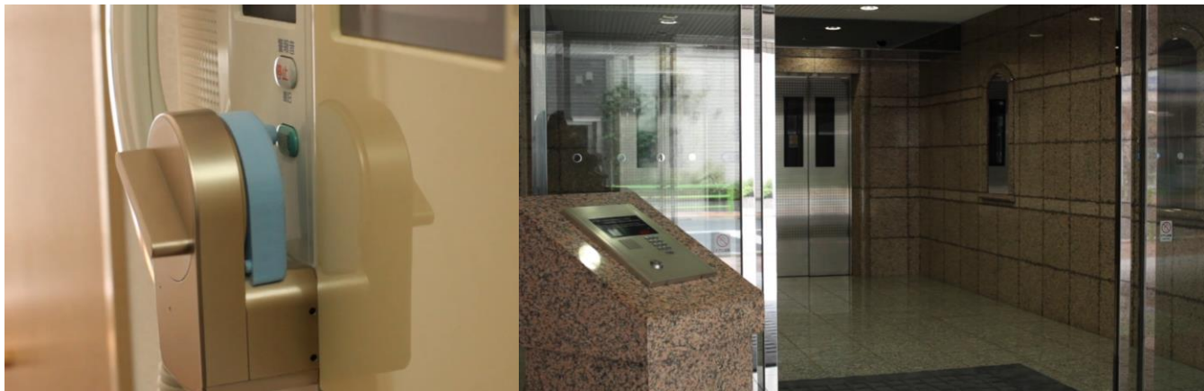
「SESAME mini」に拡張ホルダーを取り付け、玄関オートロックの開錠に使用している様子
