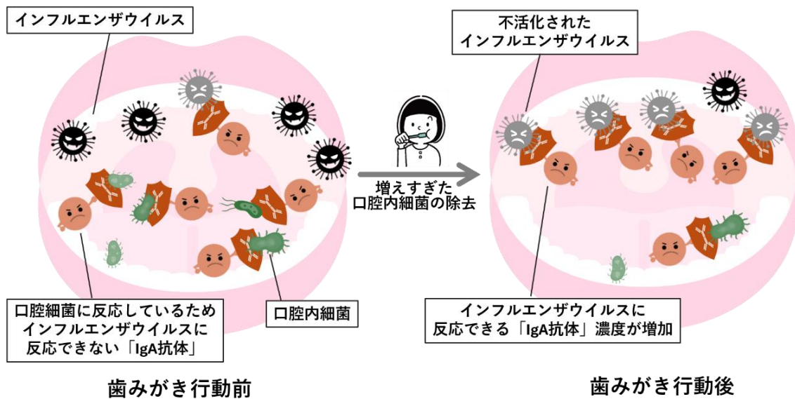
図3. 歯みがき行動によるインフルエンザウイルス不活化能向上のメカニズム考察
