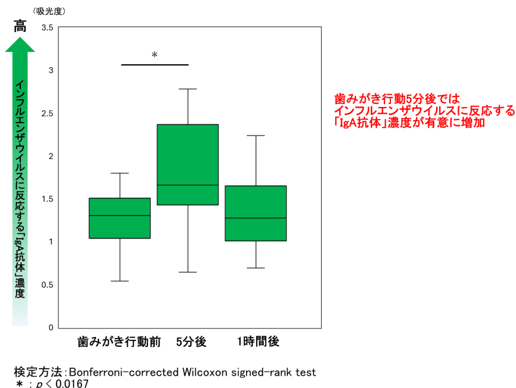
図2. 歯みがき行動前後でのインフルエンザウイルスに反応する唾液中の「IgA抗体」濃度の変化
