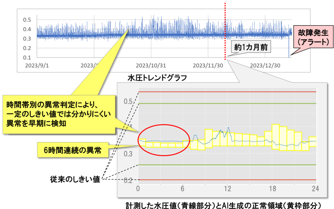
減圧弁故障の予兆検知イメージ
