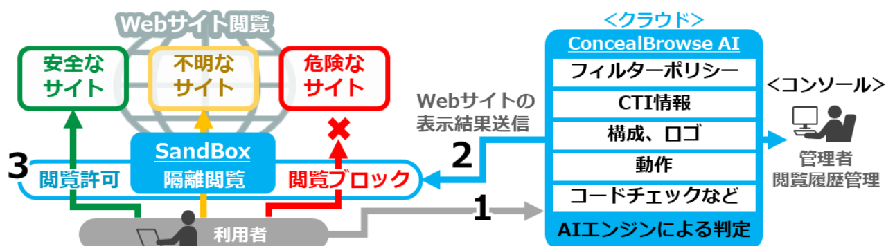
「ConcealBrowse」の機能概要
