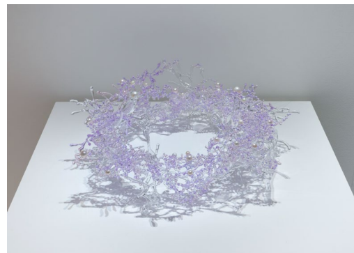
「Dequeuer-circulate」
