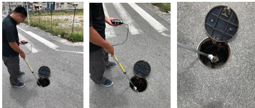
<TS リークチェッカー使用風景>
