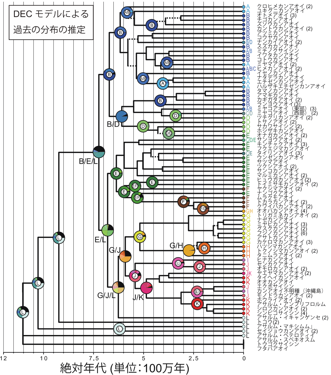
図 2 : 最尤法を用いて推定したカンアオイ類 (狭義) 54 種の系統関係。横軸は推定された分岐年代を示している。A-L は現在カンアオイが分布している地域を 12 に分割した領域を表しており (図 3 参照)、系統樹の主要な分岐点において推定される過去の分布地域を円グラフで示している。
