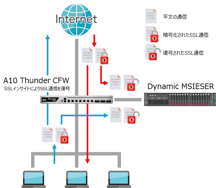
Dynamic MSIESER と A10 Thunder CFW の連携 イメージ図
