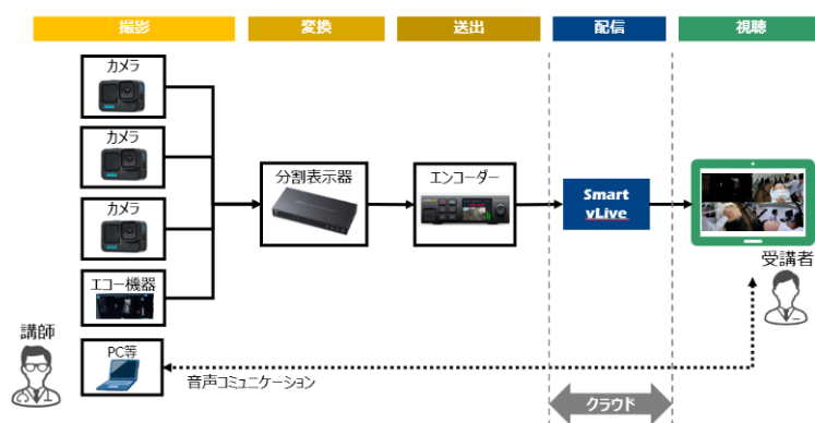
構成図
