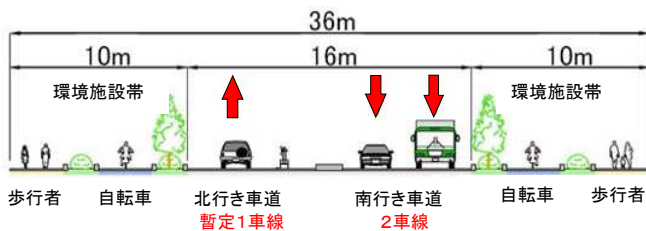
A-A'断面およびB-B'断面
