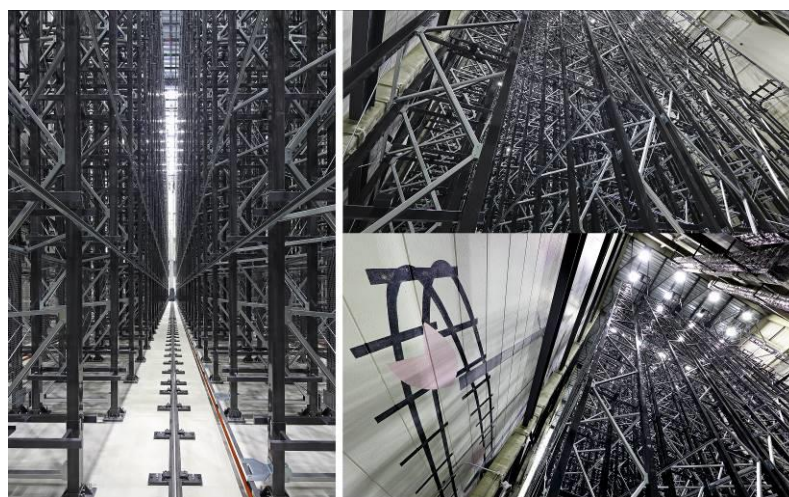
自動倉庫
