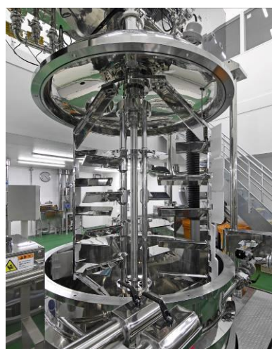
大型乳化機
